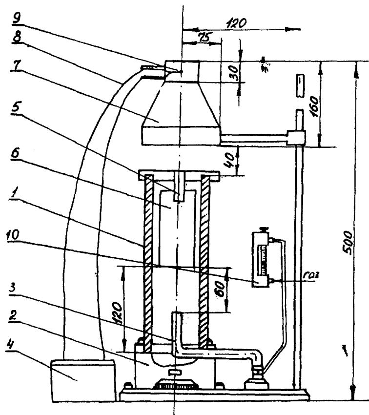
Рис. 1. Установка для определения огнезащитной эффективности ОЗСВ:
