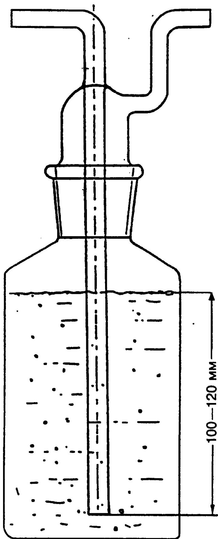
Рисунок 2 - Сосуд-смеситель
