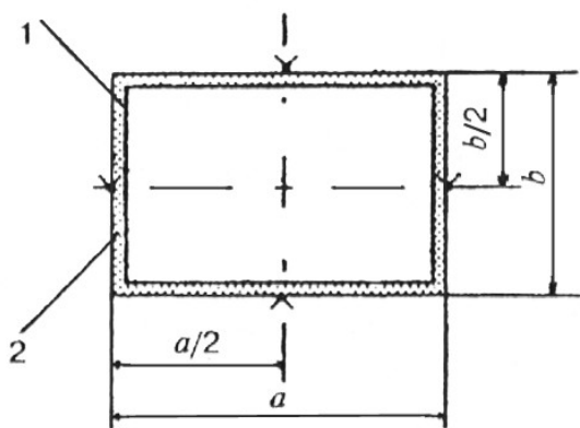
1 - воздуховод; 2 - покрытие воздуховода; \blacktriangledown - термоэлектрические преобразователи (ТЭП); a, b - размеры поперечного сечения воздуховода
