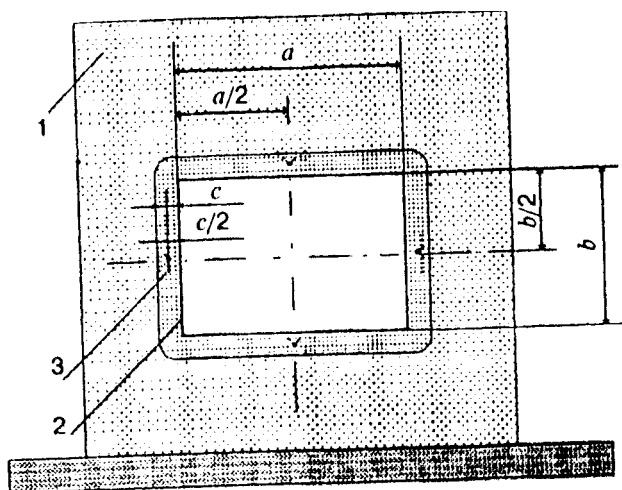
1 - печь; 2 - воздуховод, 3 - уплотнение места проходки воздуховода через ограждающую конструкцию печи; \blacktriangledown - термоэлектрические преобразователи (ТЭП); a, b - внутренние размеры поперечного сечения воздуховода, c - толщина заделки
