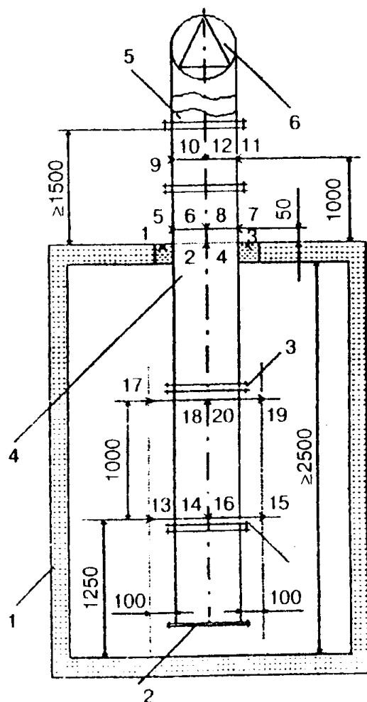
Рисунок А. 1 - Схема размещения горизонтальных воздуховодов на испытательном стенде
