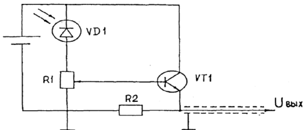
Схема электрическая принципиальная: VD1 - ФД-9К; VT1 - КТ 315Е; R1 - 1,8 кОм; R2 - 300 Ом
