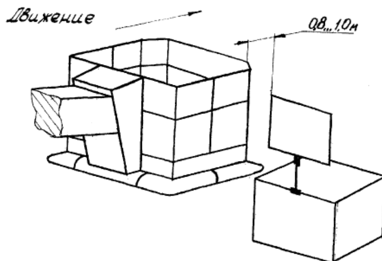
Рисунок 1. Схема положения люльки АПК относительно приспособления “щит-препятствие” при перемещении колен стрелы относительно друг друга
