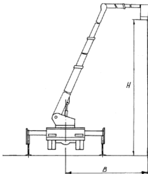
Основные технические параметры АПК: H - высота подъема; B - вылет
