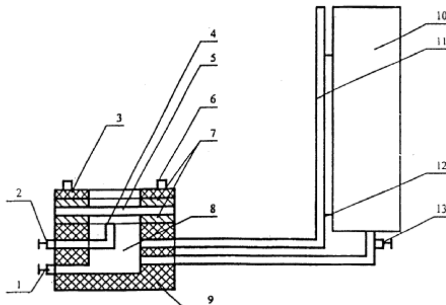
Рисунок 4. Схема установки для определения водонепроницаемости материалов (накетов) БОП-С:
