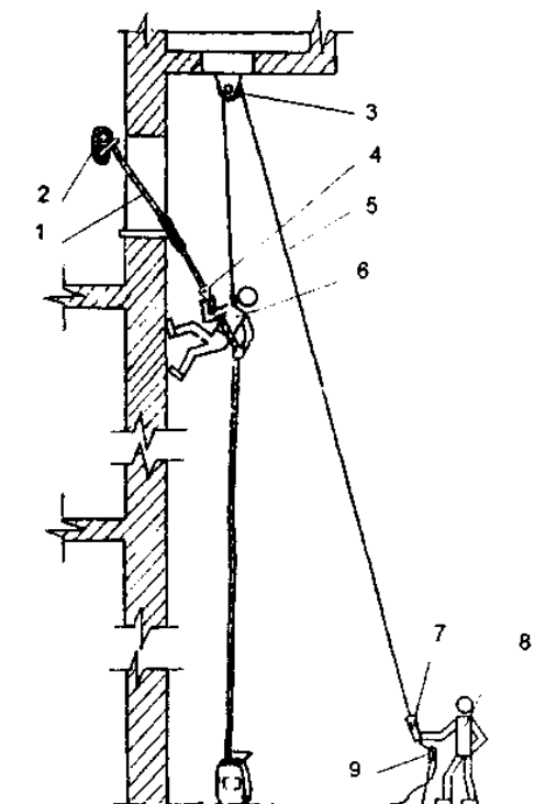
Рисунок 4. Схема страховки при спуске испытателей на УКСП:
