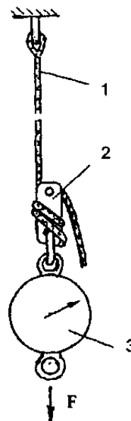
Рисунок 3. Схема нагружения УКСПр: 1 - канат; 2 - тормозное устройство; 3 - динамометр
