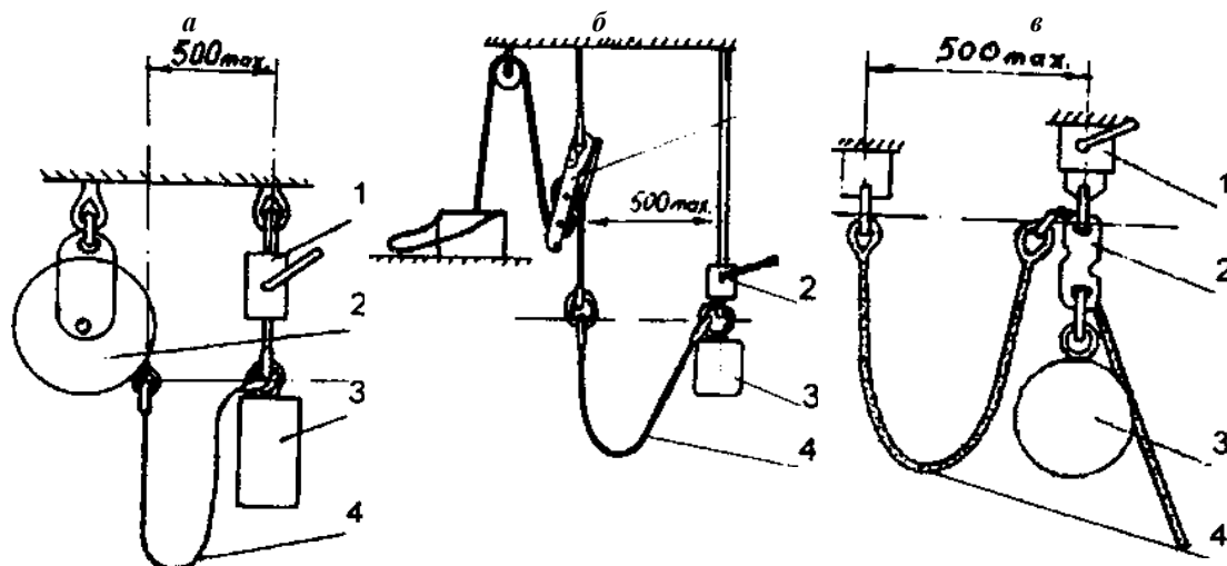
Рисунок 5. Схемы испытания УКСП на динамическую прочность: а - схема испытания УКСПа; б - схема испытания УКСПр при закреплении тормозного устройства на стенде; в - схема испытания УКСПр при закреплении тормозного устройства на контрольном грузе; 1 - расцепляющее устройство; 2 - тормозное устройство; 3 - контрольный груз; 4 - фал
