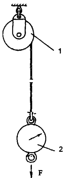
Рисунок 2. Схема нагружения УКСПа: 1 - УКСПа; 2 - динамометр
