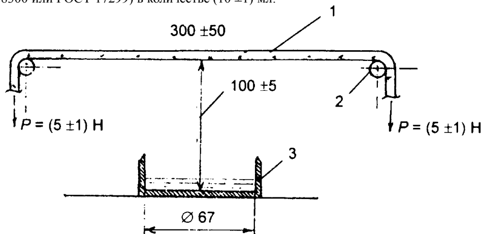
Рисунок 6. Схема стенда для испытания каната УКСП на воздействие открытого пламени: 1 - канат УКСП; 2 - опоры; 3 - емкость для горючего
