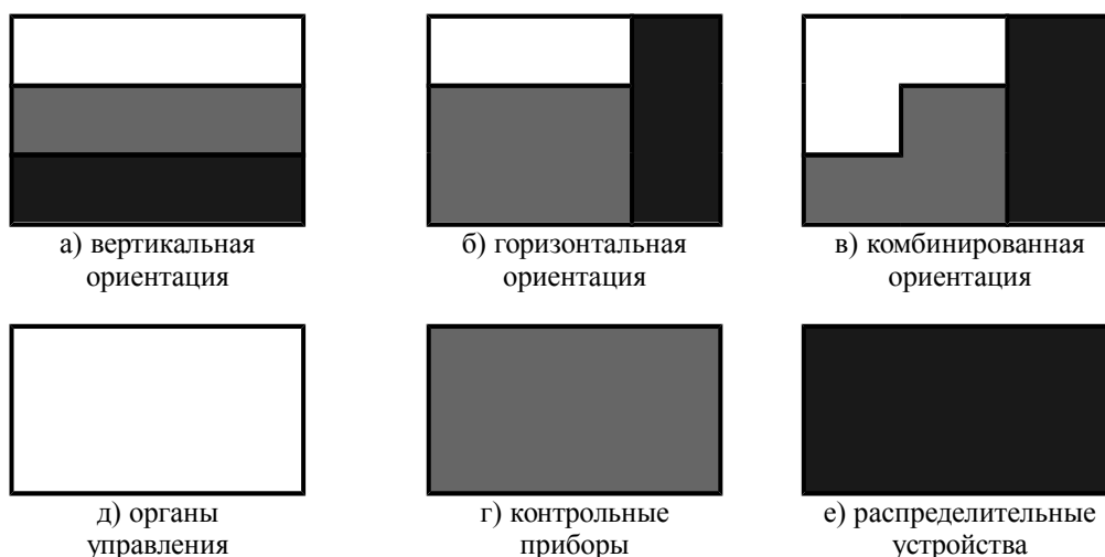
Рисунок 2. Варианты компоновки щитов управления
