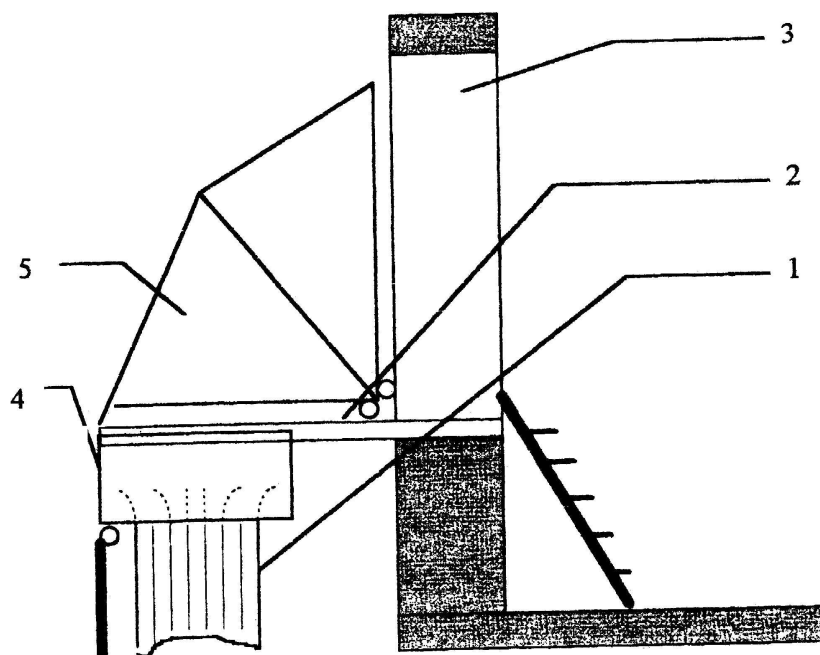
Рисунок 1. Схема рукавного пожарного спасательного устройства: 1 - спасательный рукав; 2 - узел крепления; 3 - проем стены здания; 4 - контейнер для хранения спасательного рукава; 5 - защитный тент
