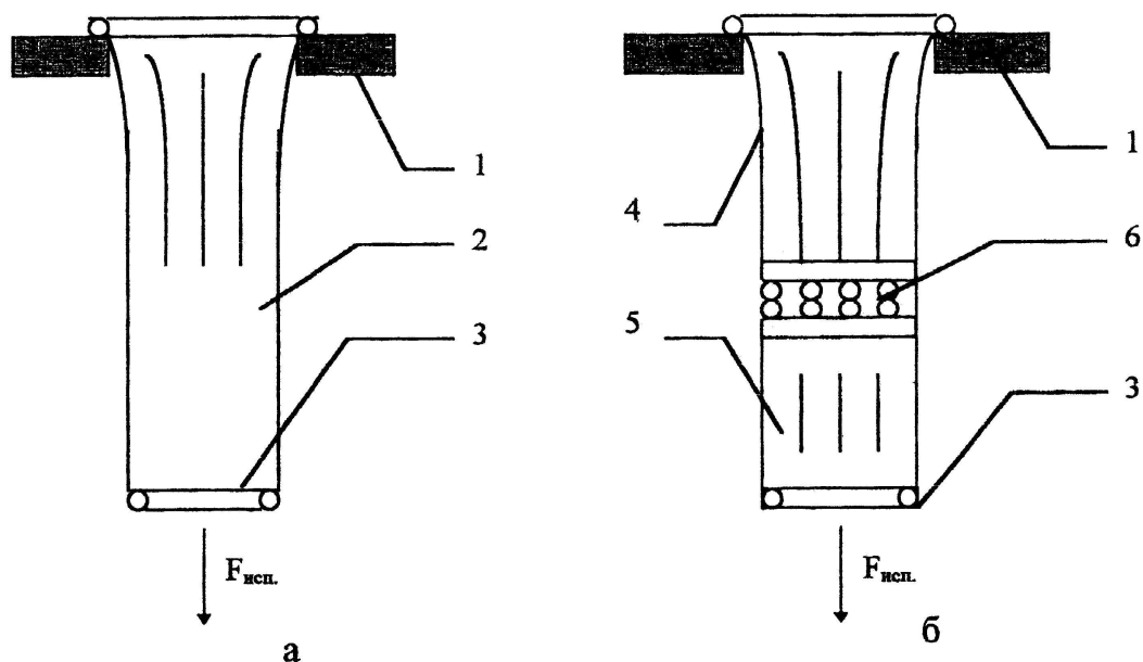
Рисунок 4. Схема испытания спасательного рукава на прочность: а - схема испытания сплошного рукава; б - схема испытания секционного рукава; 1 - верхняя траверса испытательного стенда; 2 - спасательный рукав; 3 - нижняя траверса испытательного стенда; 4 - верхняя секция; 5 - нижняя секция; 6 - узел стыковки секций спасательного рукава
