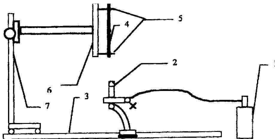
Рисунок 8. Схема установки для испытания текстильных материалов на воздействие открытого пламени:
