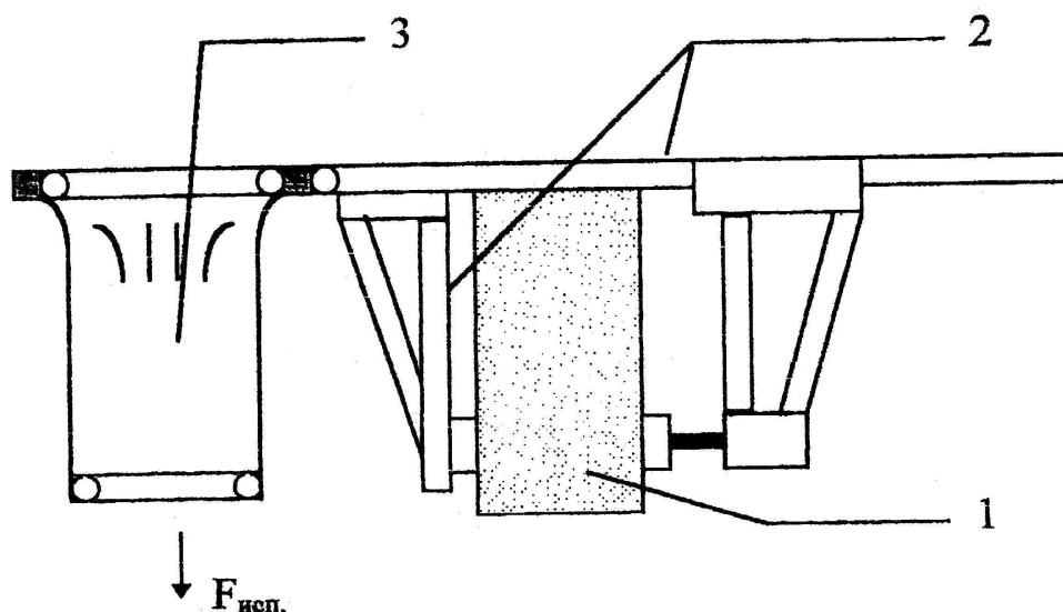
Рисунок 5. Схема испытания на прочность переносного УСРП: 1 - опора объекта или испытательного стенда; 2 - узел крепления; 3 - спасательный рукав
