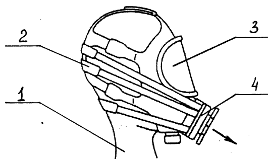
Рис. 1. Установка для определения прочности крепления соединительной коробки к лицевой части и корпуса клапана выхода к корпусу лицевой части:
