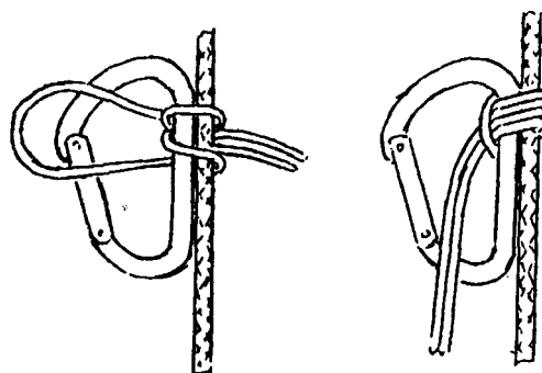
Рис. 11. Узел Бахмана
