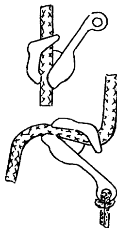
Рис. 9. Зажим Хиблвра
