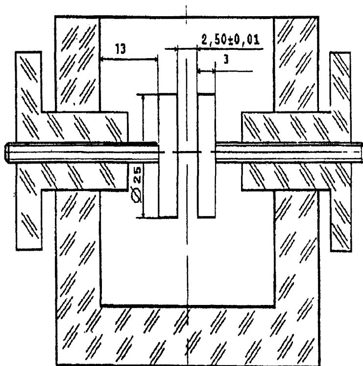
Рис. 2. Основные размеры ячейки
