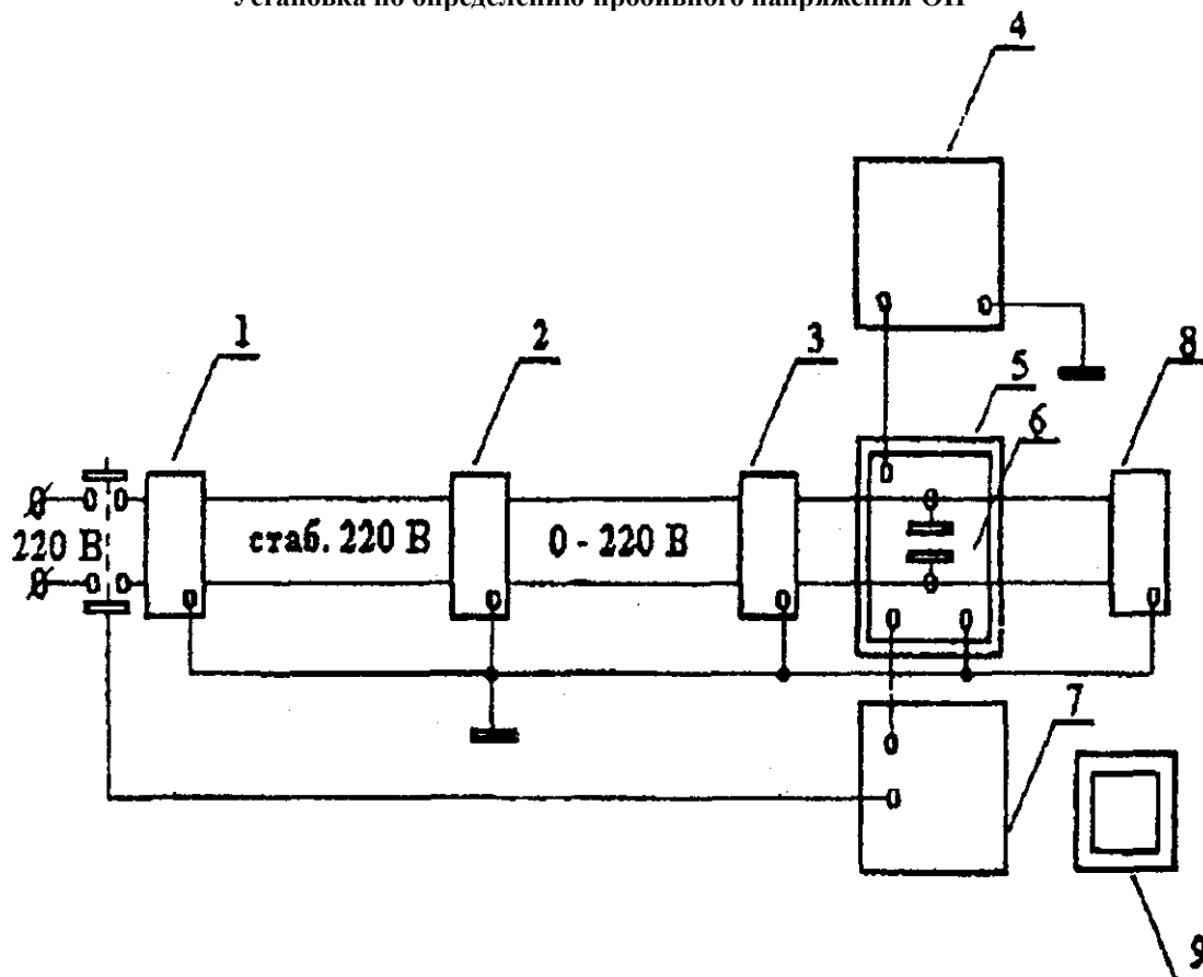
Рис. 1. Рекомендуемая блок-схема установки по определению электрической прочности огнетушащих порошков:
