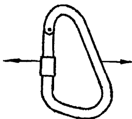
Рис. 3. Схема погружения карабина вдоль малой оси
