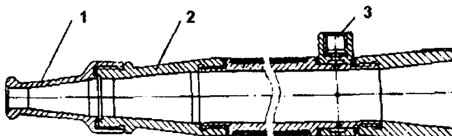
Рис. 2.1. Ствол-водомер:
