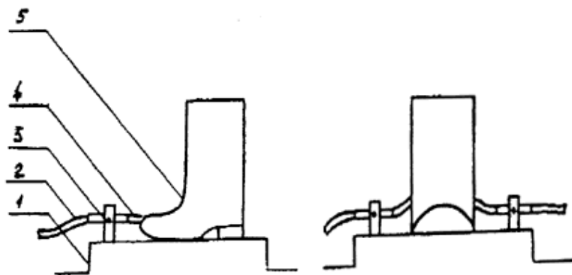
Схема установки по проверке огнезащитных свойств резиновой обуви: 1 — станина; 2 — трубка подачи газа; 3 — горелка; 4 — открытое пламя, 5 — спецобувь
