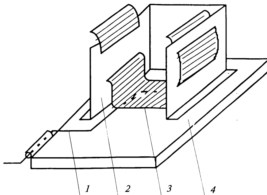
Рис. 2. Держатель с образцом: 1- термоэлектрический преобразователь, 2 - держатель, 3- исследуемый образец, 4 - керамическая пластина
