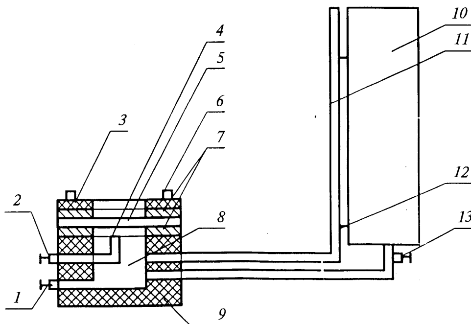
Рис. 3. Схема установки для определения водонепроницаемости материалов (пакетов) БОП: 1 - сливной кран; 2 - кран для удаления воздуха из испытательной камеры; 3 - кольцо для зажима образца; 4 - трубка для определения уровня воды в испытательной камере и слива; 5 - образец; 6 - "барашки"; 7 - резиновые прокладки; 8 - испытательная камера; 9 - основание камеры; 10 - емкость с водой, создающая давление на образец; 11 - трубка со шкалой делений для измерения давления на образец; 12 - крепление трубки со шкалой делений к емкости с водой; 13 - кран подачи воды в испытательную камеру
