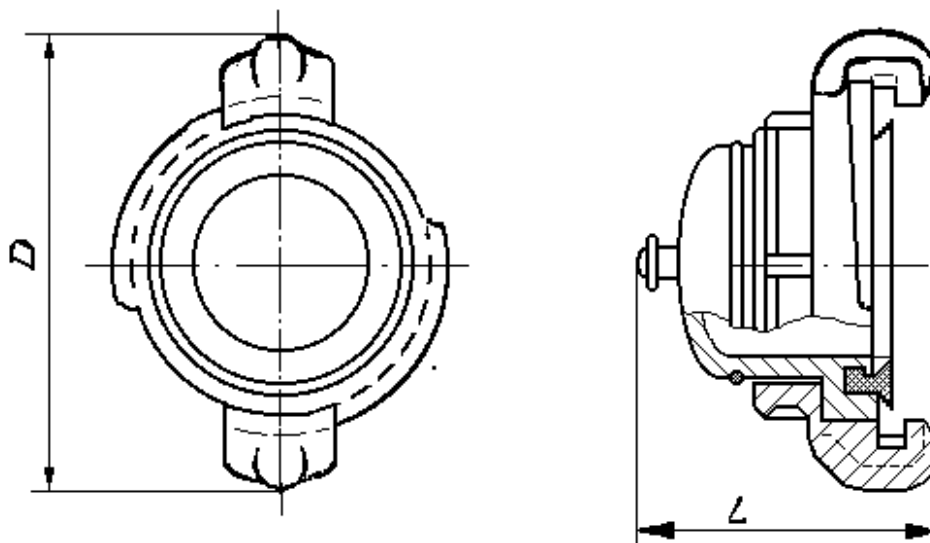
Рисунок 8. Всасывающая головка-заглушка
