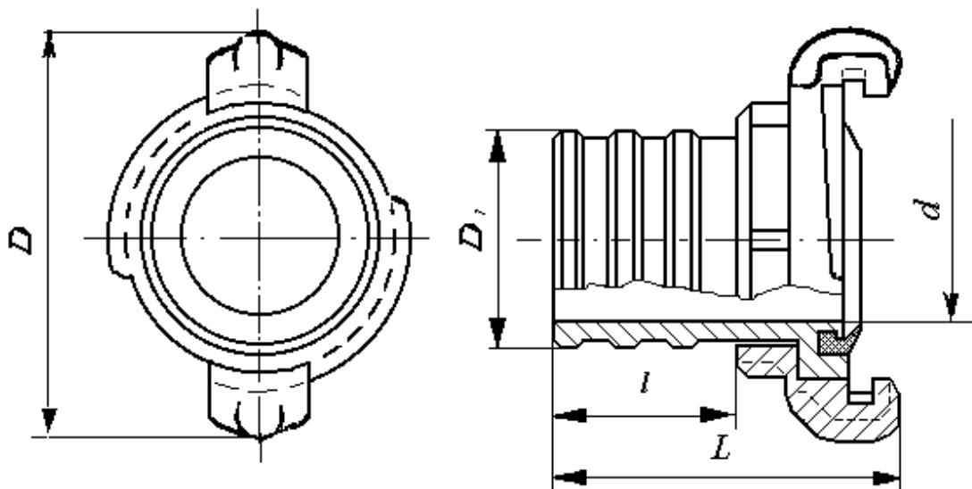
Рисунок 1. Рукавная напорная головка
