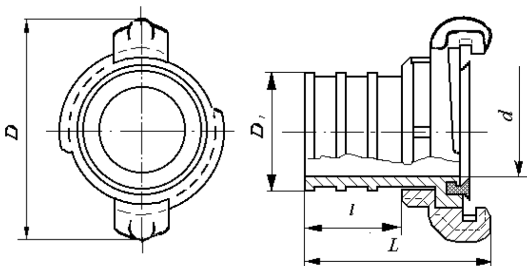
Рисунок 6. Рукавная всасывающая головка
