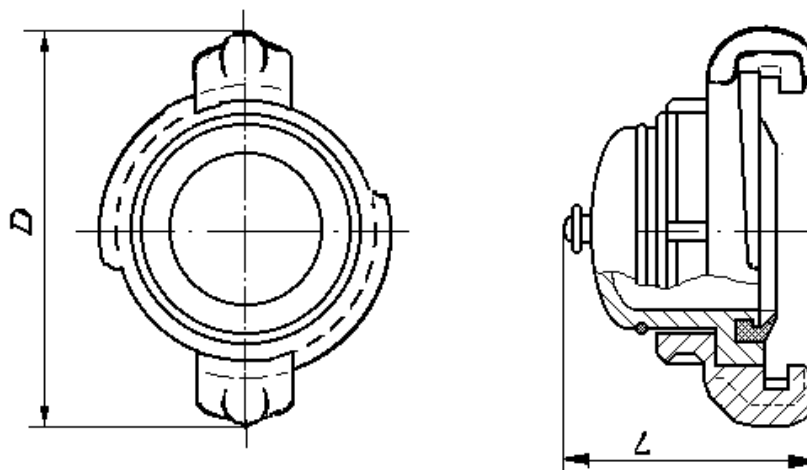
Рисунок 5. Напорная головка-заглушка
