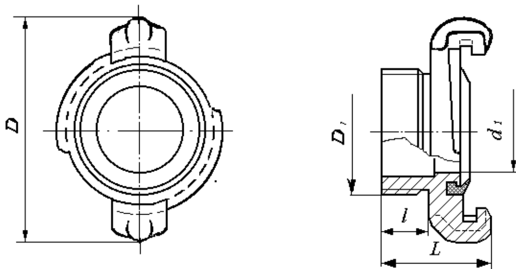
Рисунок 3. Цапковая напорная головка
