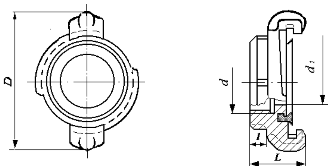
Рисунок 7. Муфтовая всасывающая головка
