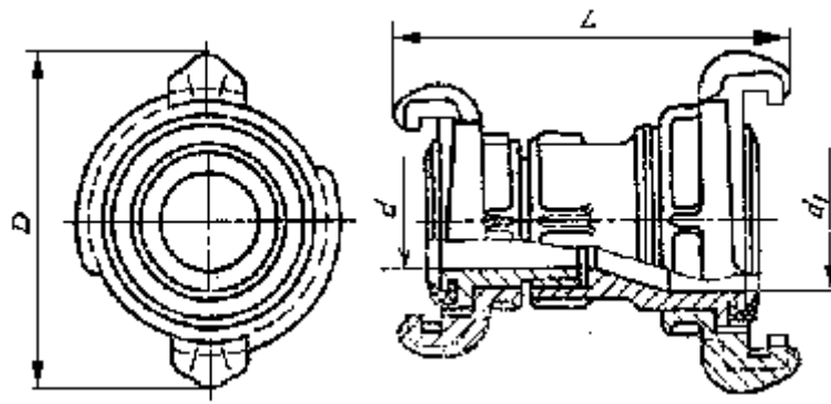
Рисунок 4. Переходная напорная головка
