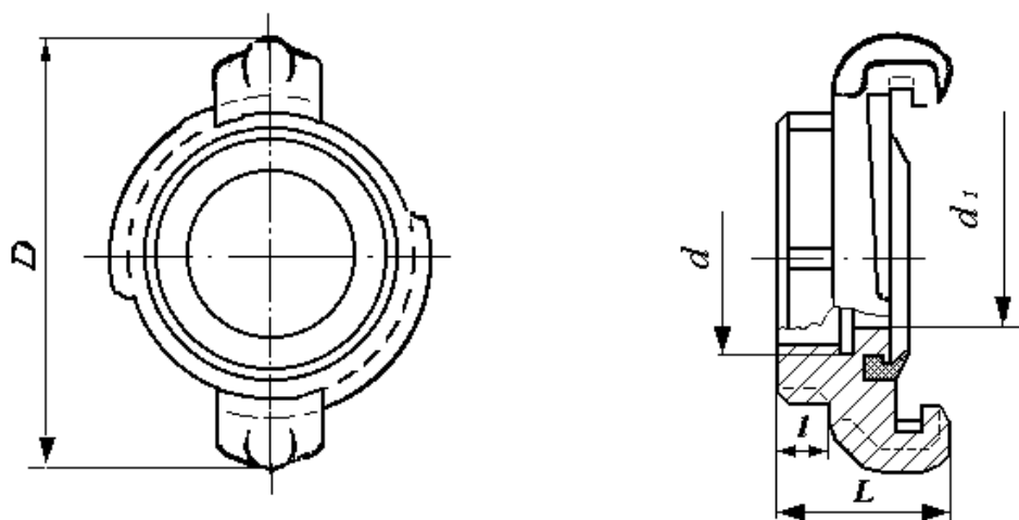
Рисунок 2. Муфтовая напорная головка
