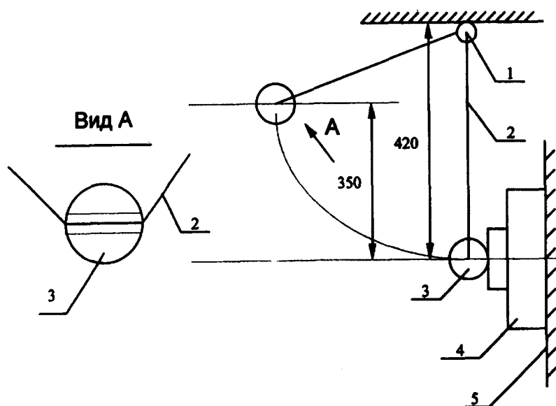
1 - горизонтальная штанга; 2 - нить маятника; 3 - латунный шар; 4 - испытуемый шар; 5 - опора
