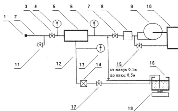
Рис.1. Схема установки для испытаний пеносмесителей (дозаторов):
