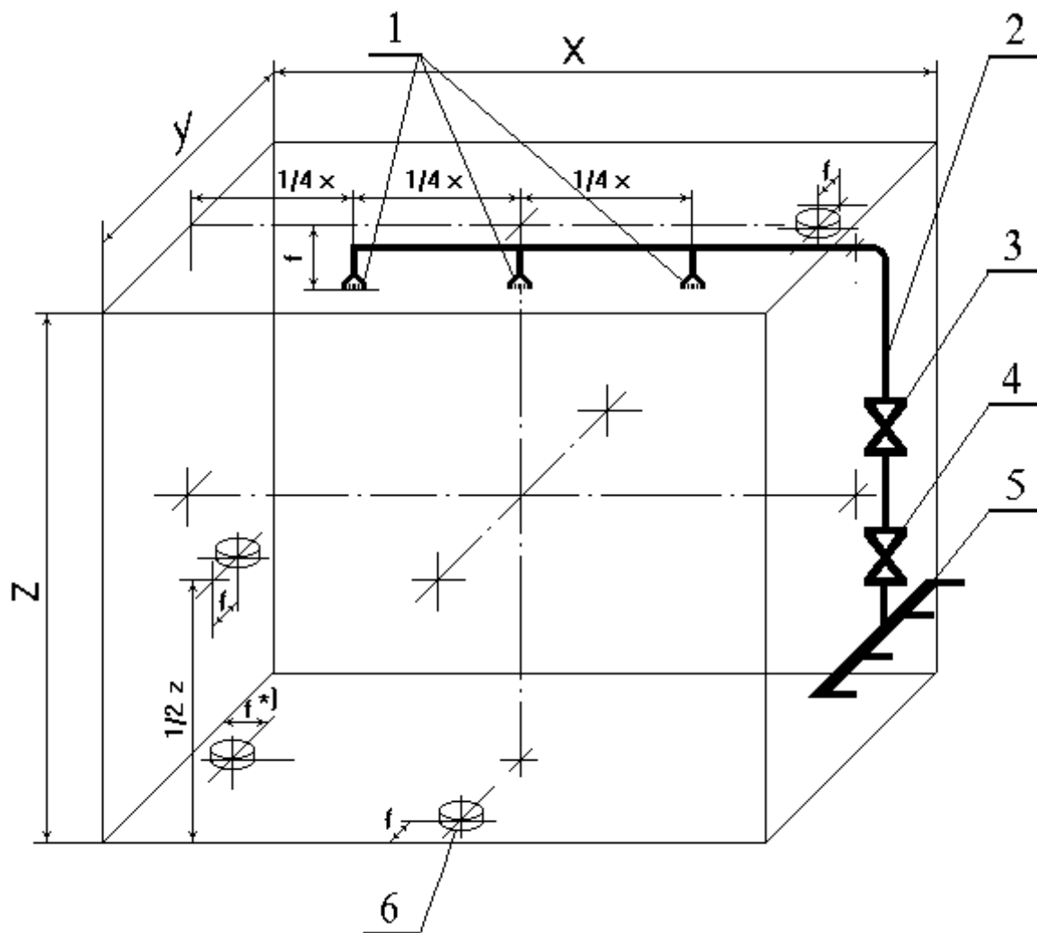
Рис. 2. Схема расположения газовой арматуры и горелок в огневой камере: 1 - газовые насадки; 2 - трубопровод; 3 - запорный клапан; 4 - регулирующий клапан; 5 - коллектор; 6 - горелка
