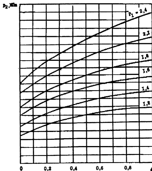
Рис. 1. График для определения давления в изотермической емкости в конце выпуска расчетного количества двуокиси углерода.
