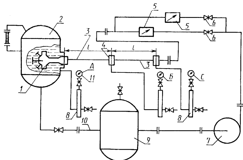
1 — испытуемое изделие; 2 — основной бак; 3 — мерный участок трубопровода; 4 — уравнивающая камера; 5 — расходомер; 6 — задвижка; 7 — центробежный насос; 8 — демпферное устройство; 9 — кавитационный бак; 10 — трубопровод; 11 — манометр. Черт. 2
