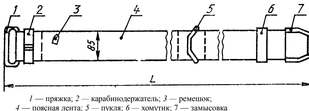
Рисунок 2. Пояс без амортизирующего устройства (тип Б)
