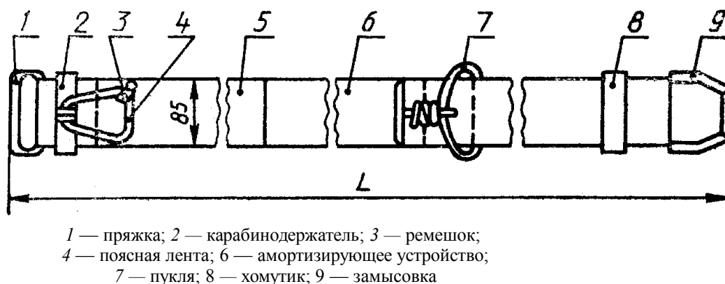
Рисунок 1. Пояс с амортизирующим устройством (тип А)
