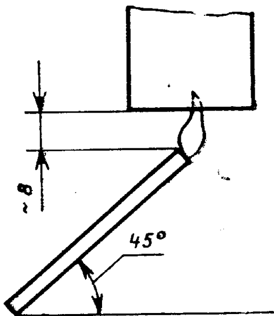
Испытательный образец Черт. 2
