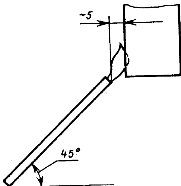
Испытательный образец Черт. 3
