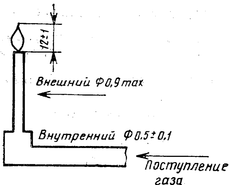
Поступление газа Черт. 1
