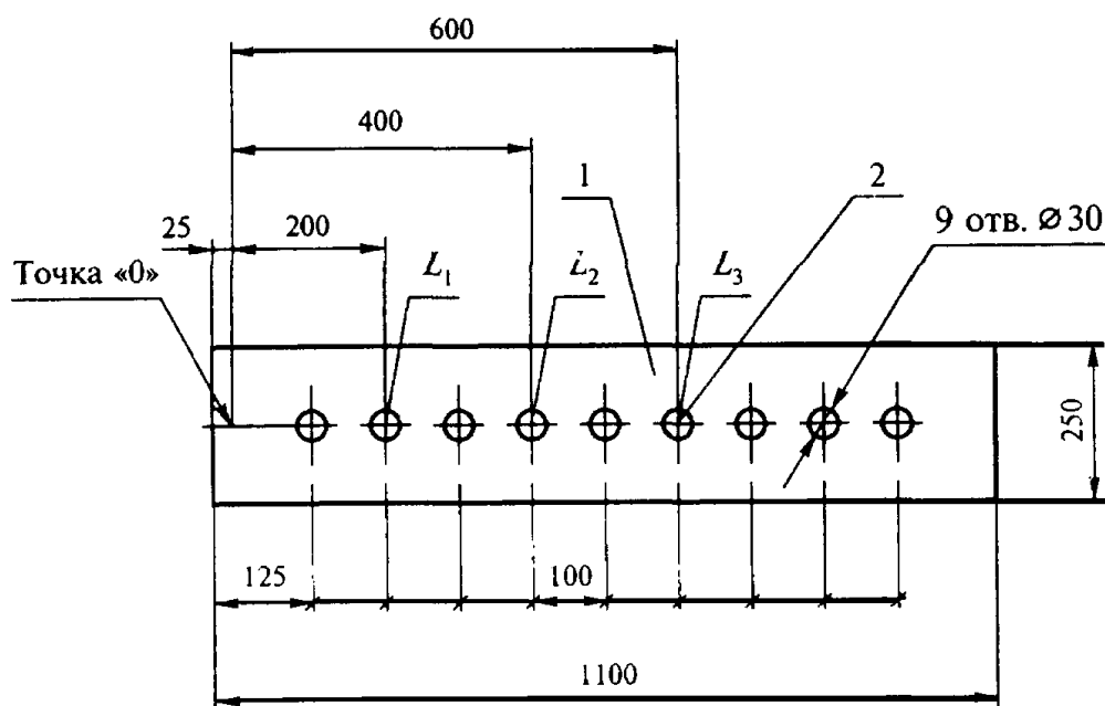
Рисунок 4 -Калибровочный образец
