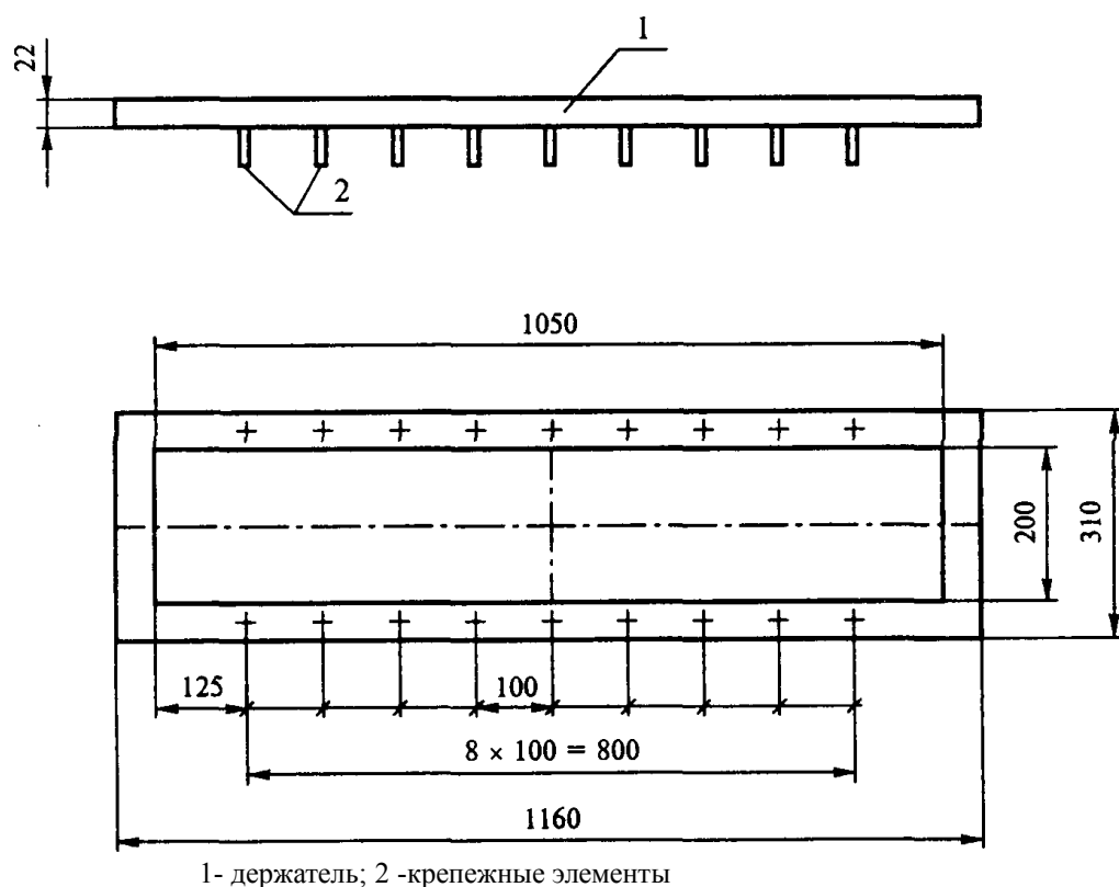
Рисунок 3 -Держатель образца
