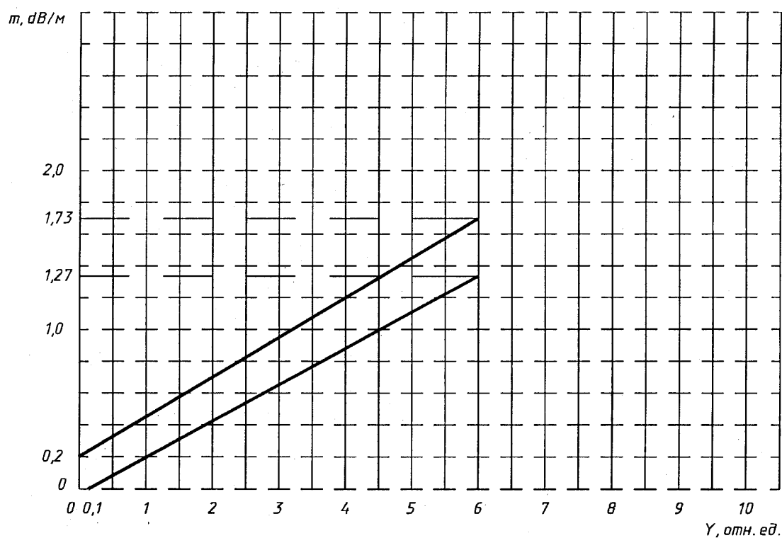
Рисунок Л.8 - Тестовый очаг пожара ТП-4. Зависимость оптической плотности от концентрации продуктов горения
