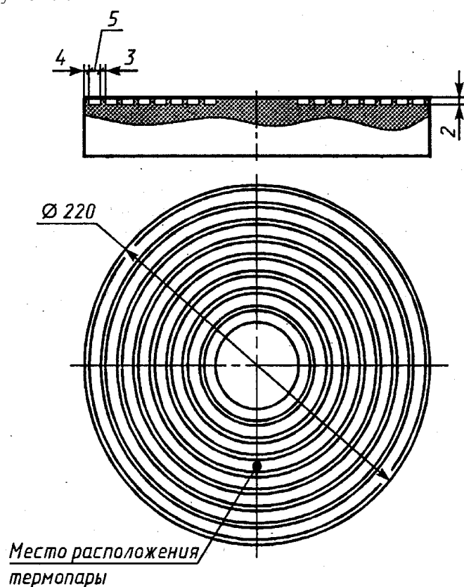
Рисунок В.1 — Внешний вид рабочей поверхности электроплиты
