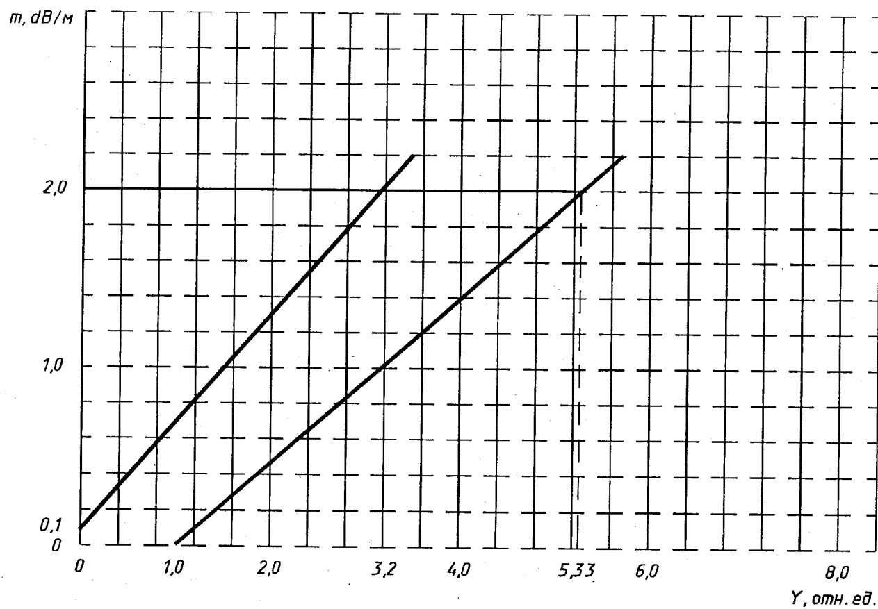
Рисунок Л.6 - Тестовый очаг пожара ТП-3. Зависимость оптической плотности от концентрации продуктов горения
