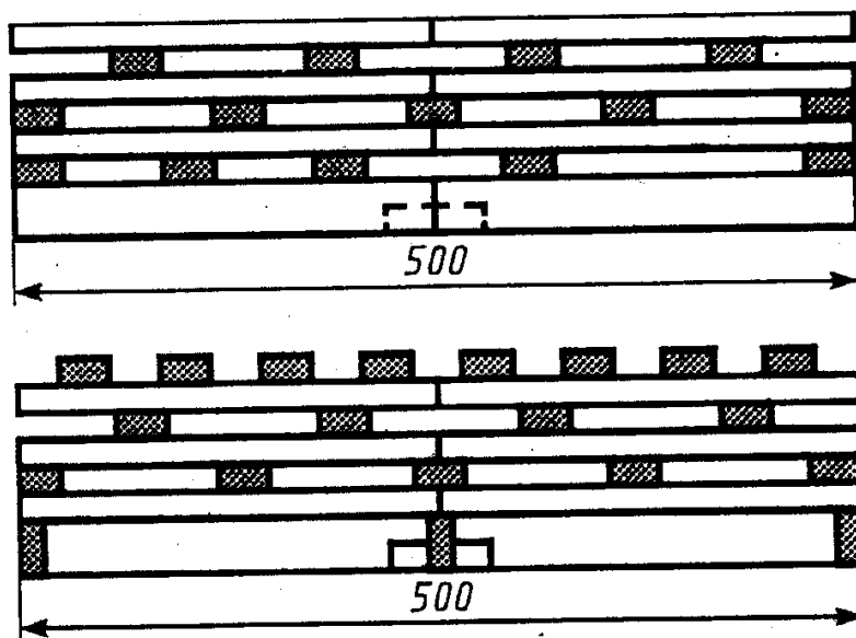
Рисунок Б.1 — Расположение буковых брусков для проведения испытаний
