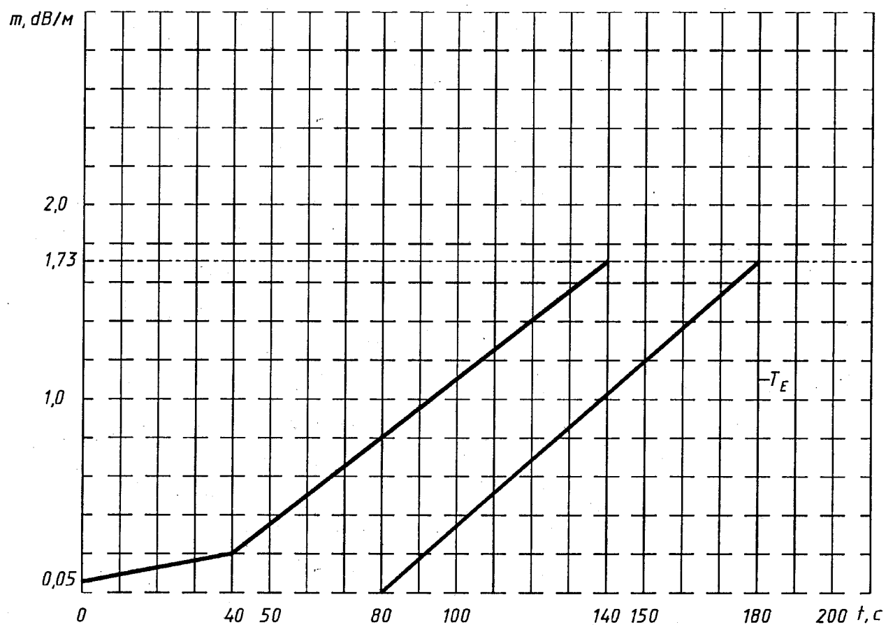
Рисунок Л.7 - Тестовый очаг пожара ТП-4. Зависимость оптической плотности среды от времени
