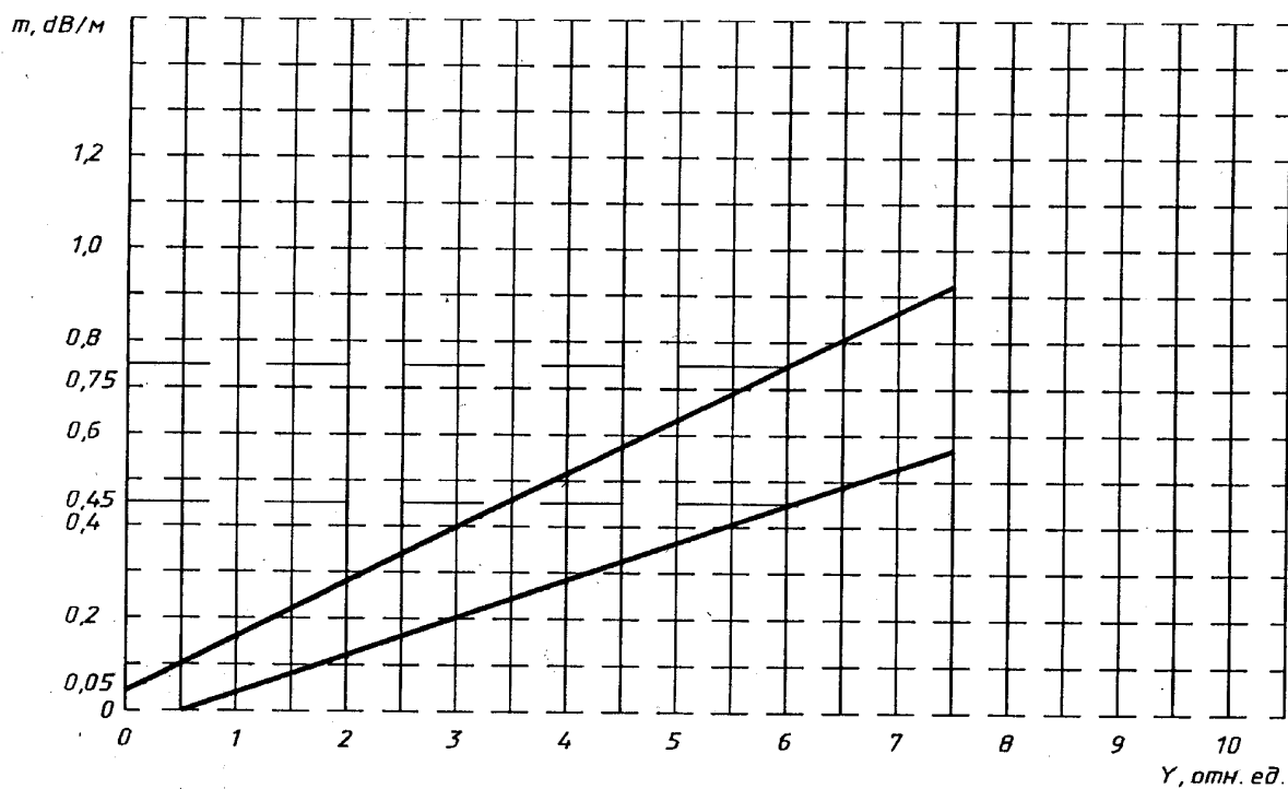
Рисунок Л.2 - Тестовый очаг пожара ТП-1. Зависимость оптической плотности от концентрации продуктов горения
