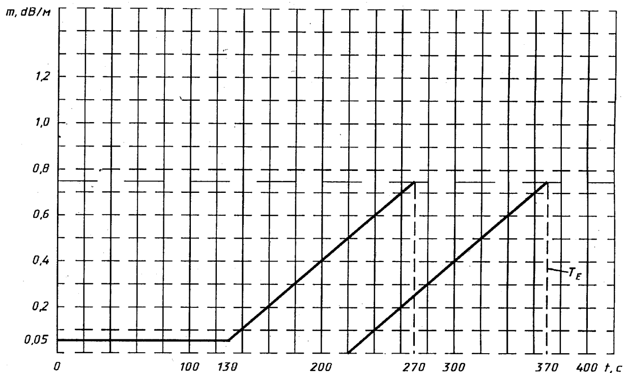
Рисунок Л.1 - Тестовый очаг пожара ТП-1. Зависимость оптической плотности среды от времени
