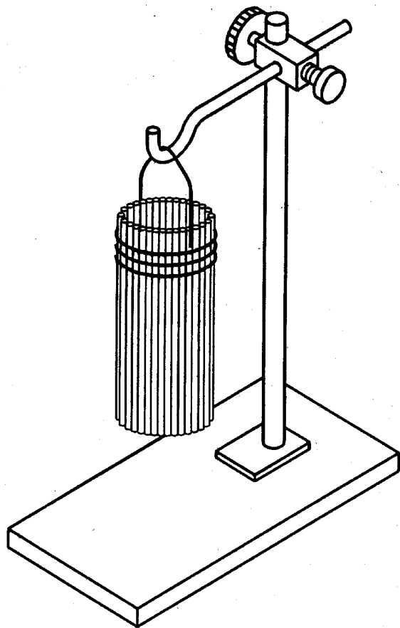
Рисунок Г.1 — Расположение хлопковых фитилей при проведении испытаний на чувствительность к тестовому очагу пожара ТП-3
