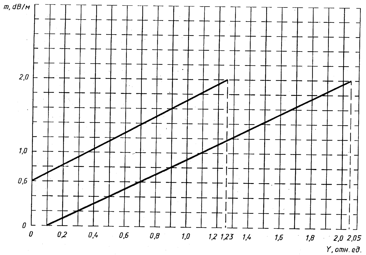
Рисунок Л.4 - Тестовый очаг пожара ТП-2. Зависимость оптической плотности от концентрации продуктов горения
