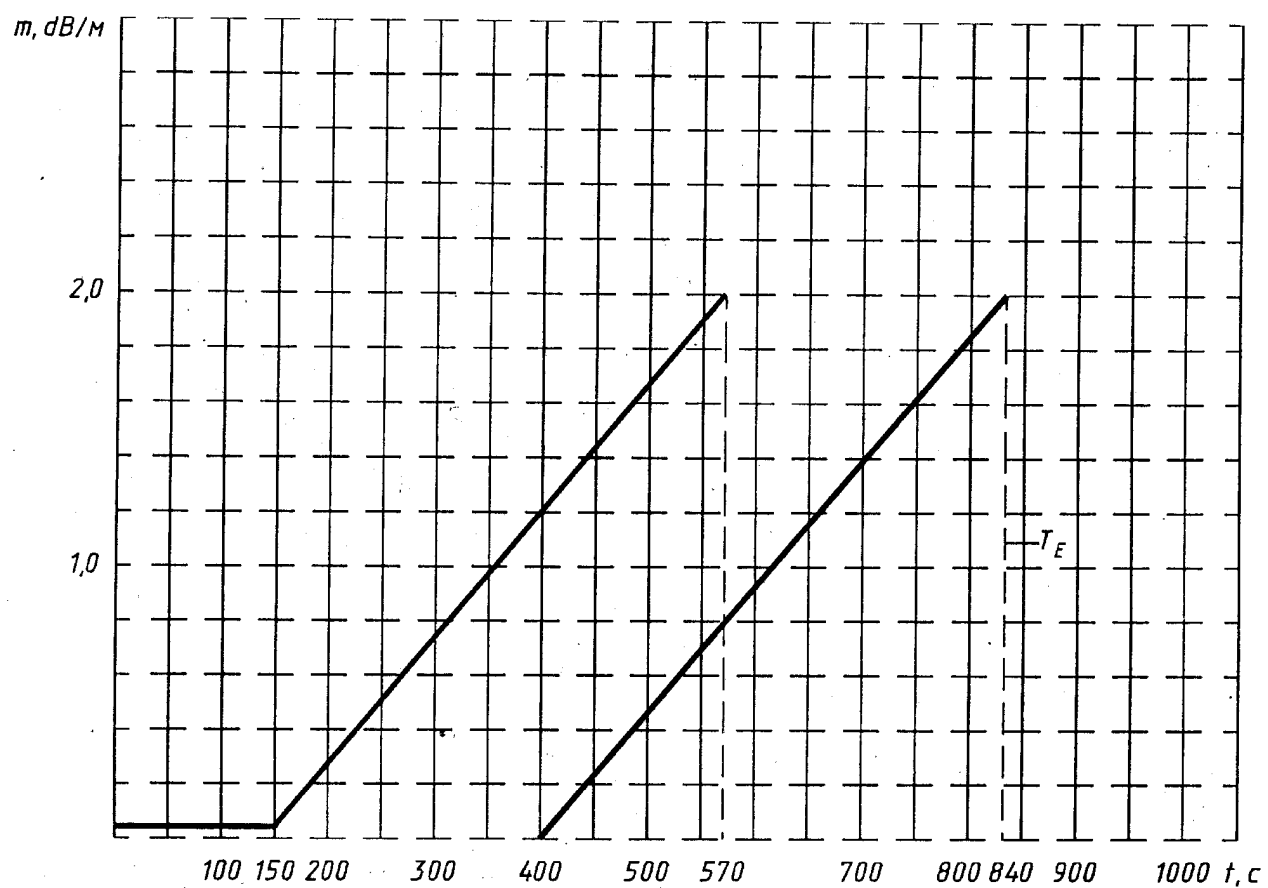
Рисунок Л.3 - Тестовый очаг пожара ТП-2. Зависимость оптической плотности среды от времени
