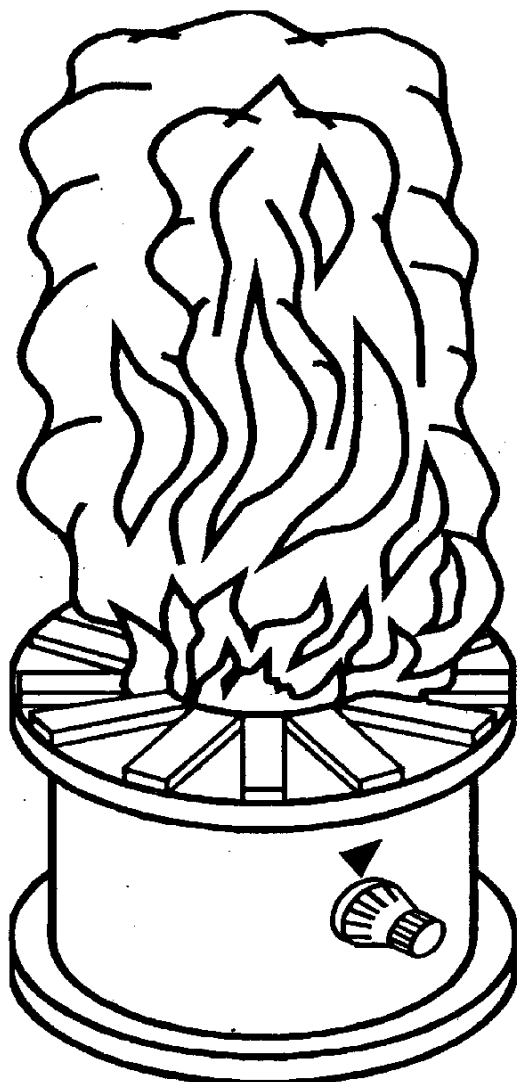
Рисунок В.2 — Расположение буковых брусков при проведении испытаний на чувствительность к тестовому очагу пожара ТП-2.
