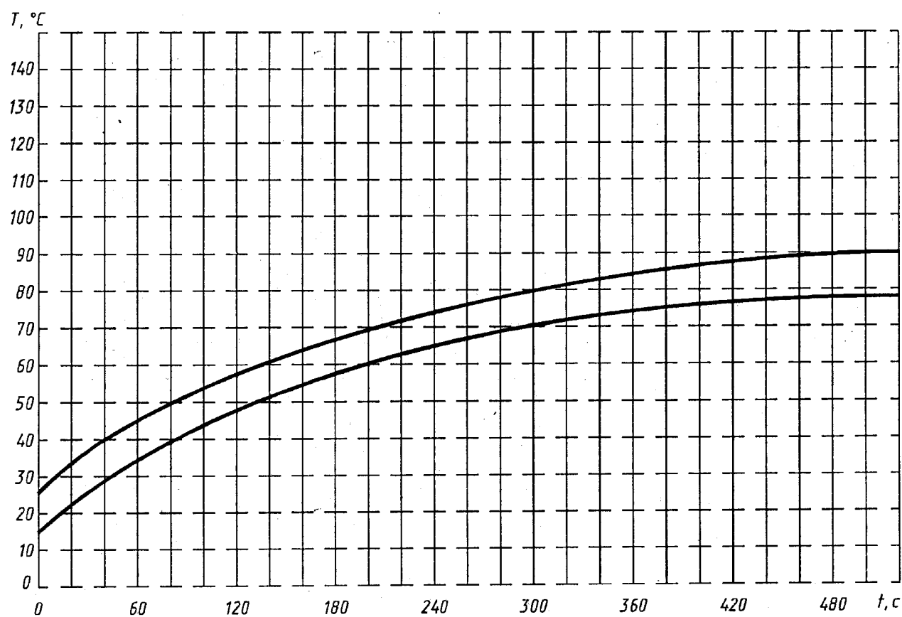
Рисунок Л.11 - Тестовый очаг пожара ТП-6. Зависимость температуры от времени
