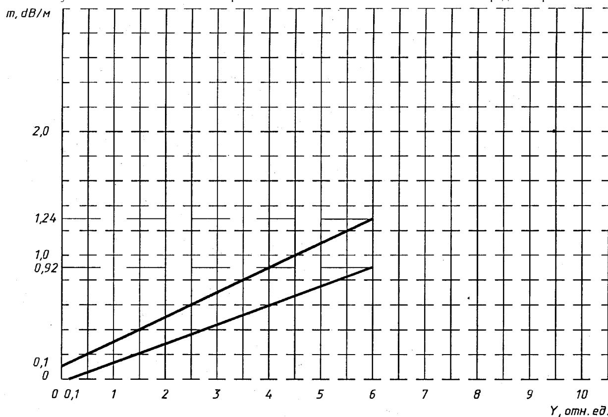
Рисунок Л.10 - Тестовый очаг пожара ТП-5. Зависимость оптической плотности от концентрации продуктов горения
