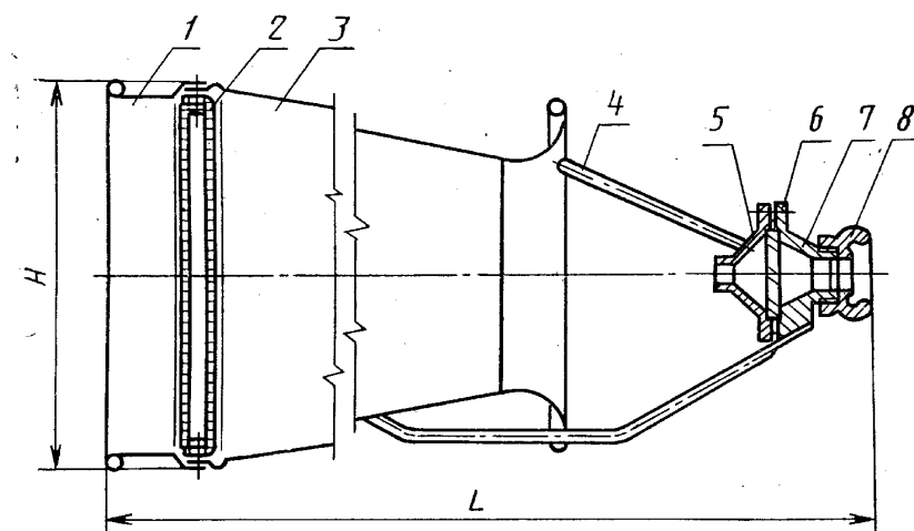
1—насадок; 2—кассета сеток; 3— корпус генератора; 4— стойка (ручка); 5—сопло; 6—распылитель; 7—корпус распылителя; 8— соединительная головка ГМ-80
