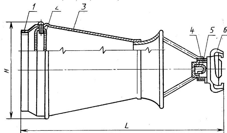
Генераторы средней кратности ГПС - 200
