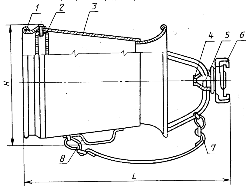
Генератор пены средней кратности ГПС-600
