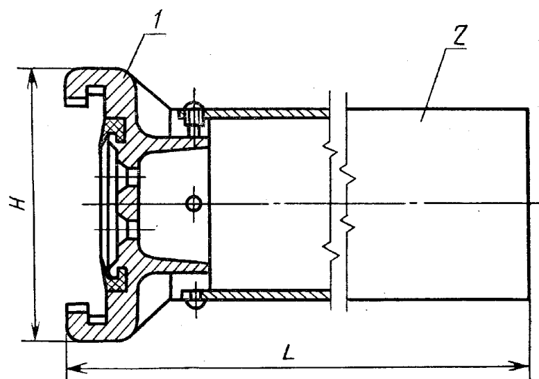
Ствол СВП
