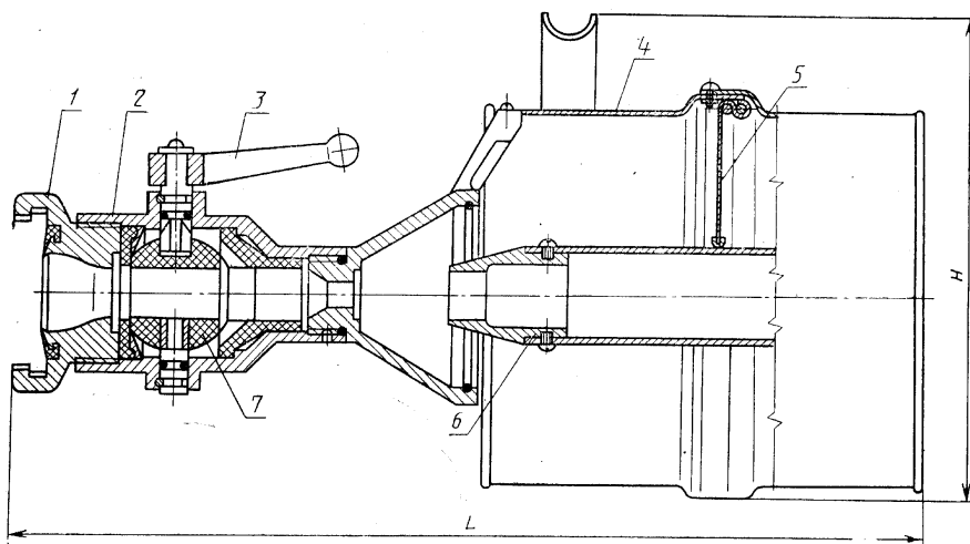
1 - соединительная головка; 2 - корпус ствола; 3 - ручка; 4 - обечайка; 5 - кассета сетки; 6 - насадок; 7 - перекрывающее устройство
