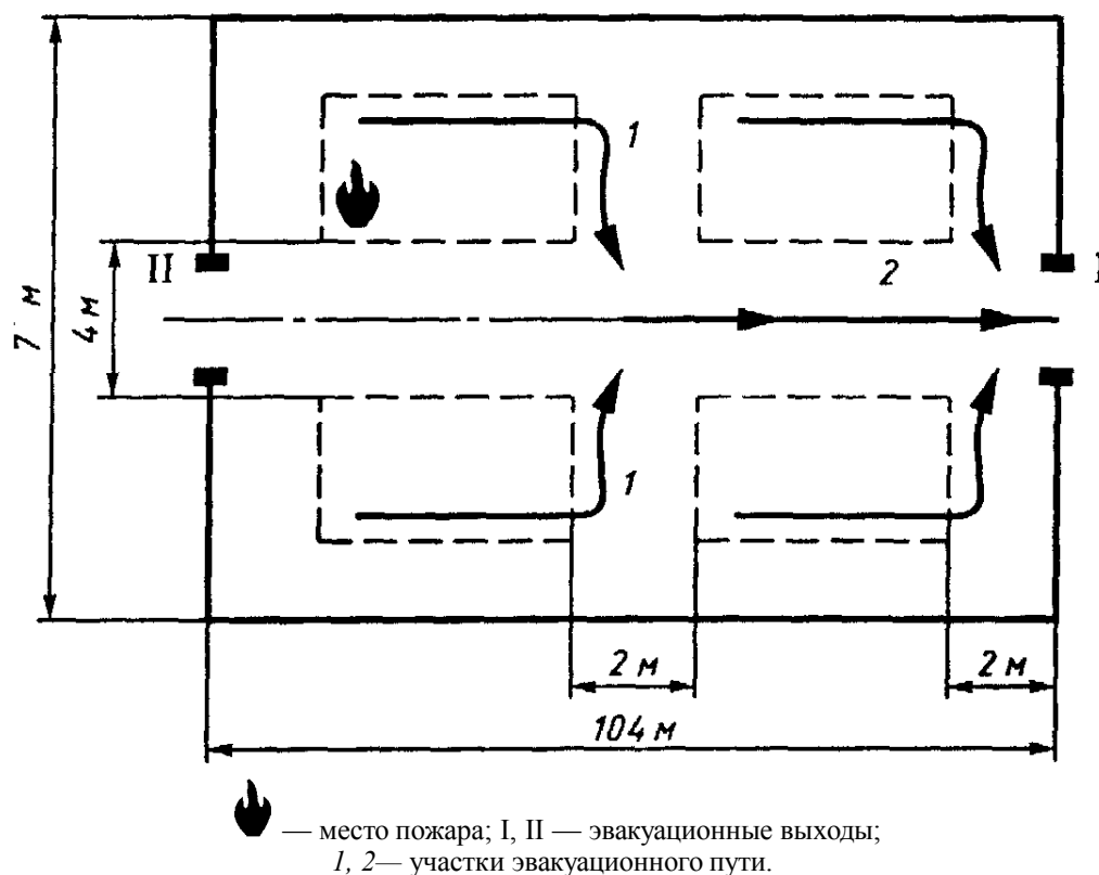
Рисунок III.2 — Расчетная схема эвакуации
