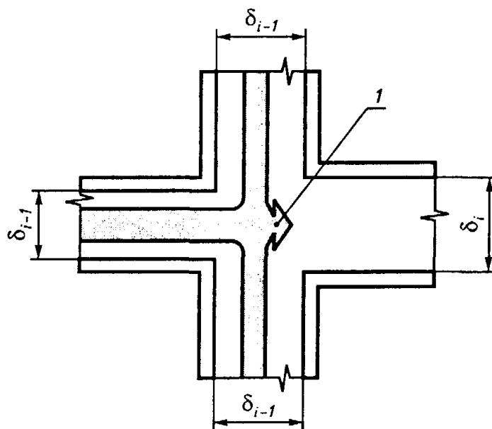
1 — начало участка i Рисунок Ш.1— Слияние людских потоков
