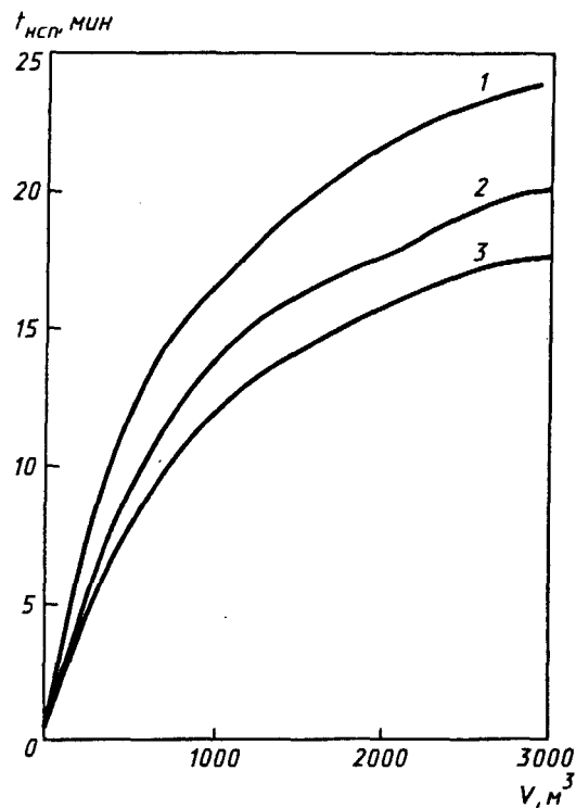
Рисунок Л.2 — Зависимость минимальной продолжительности начальной стадии пожара t_{нсп} от объема V высоты H помещения
