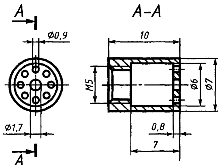
Рисунок А.4 — Схема стабилизатора пламени
