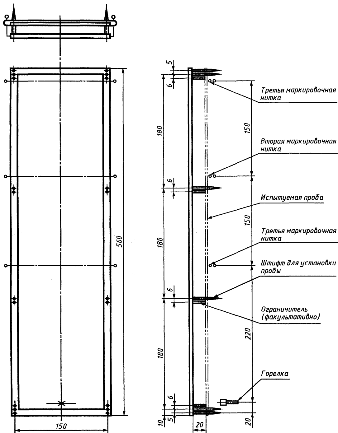
Рисунок 1 — Схема держателя для элементарной пробы
