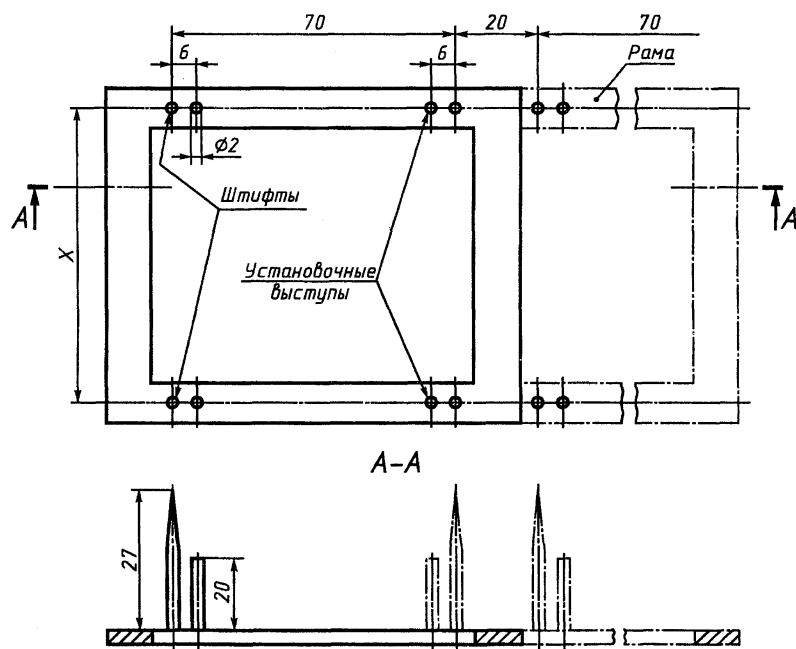
Рисунок 1 — Держатель для элементарной пробы
