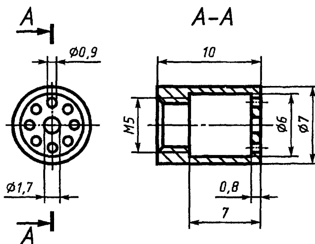
Рисунок Б.4 — Стабилизатор пламени
