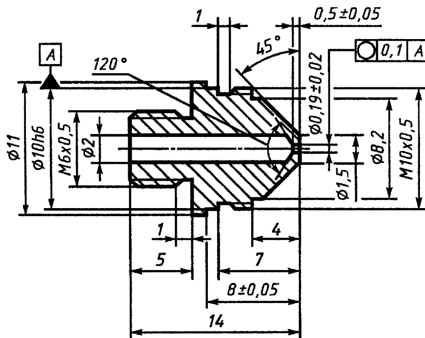
Рисунок Б.2 — Газовая форсунка
