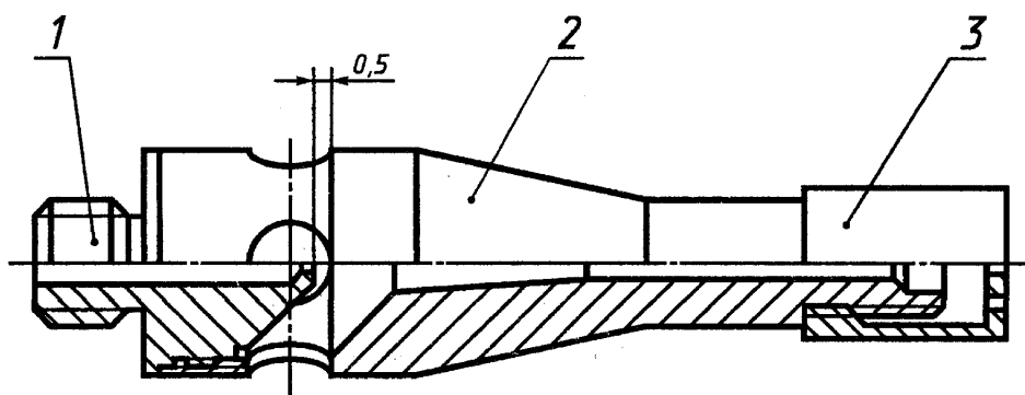
1 — газовая форсунка; 2 — трубка горелки; 3 — стабилизатор пламени
