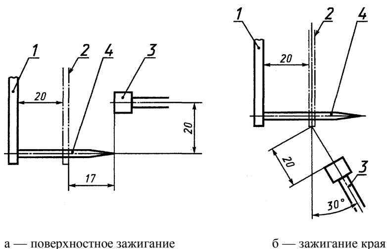
а — поверхностное зажигание б — зажигание края 1 — рама держателя; 2 — элементарная проба; 3 — горелка; 4 — штифт
