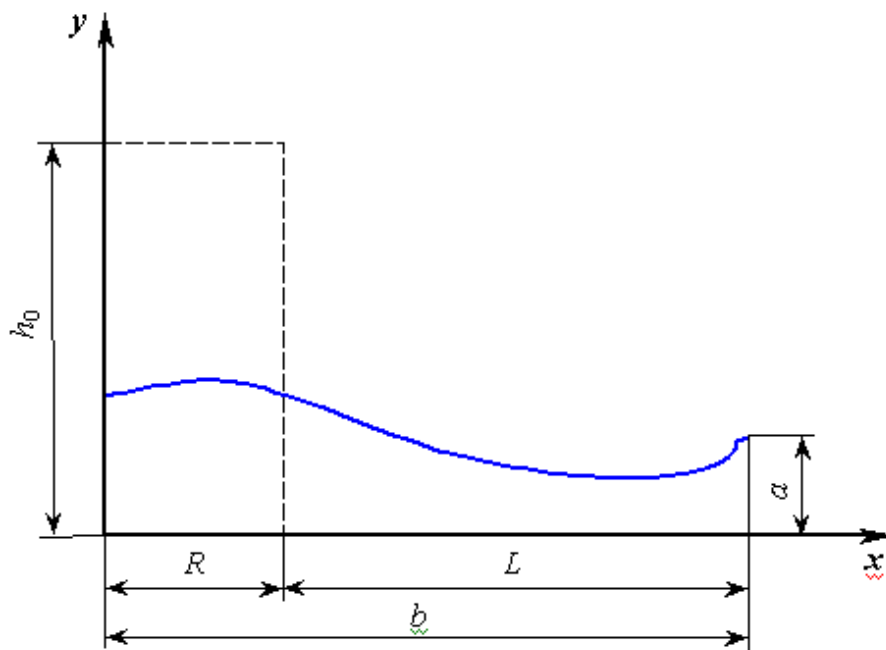
Рис.П3.2. Типичная картина движения жидкости в обваловании при квазимгновенном разрушении резервуара
