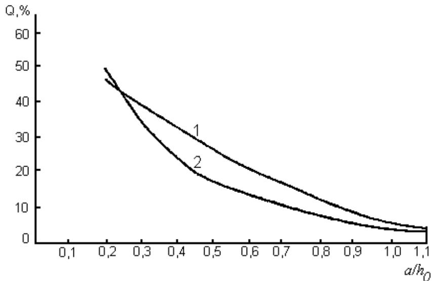
Рис.П3.3. Зависимость доли перелившейся через обвалование жидкости
