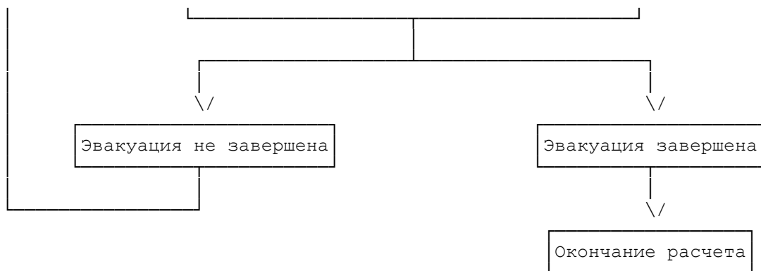
Рис. П3.2. Блок-схема определения расчетного времени эвакуации людей из здания
