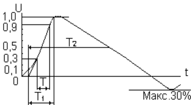
Кривая напряжения короткого замыкания (8/20 мкс)
