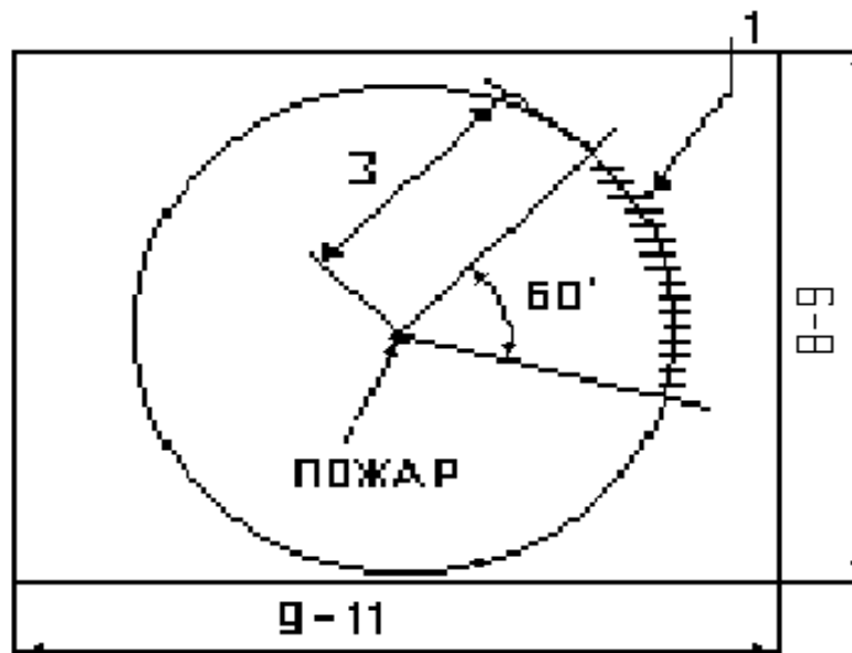
Рис. 11. Вид сверху: извещатель, очаг пожара, измерительная аппаратура.
