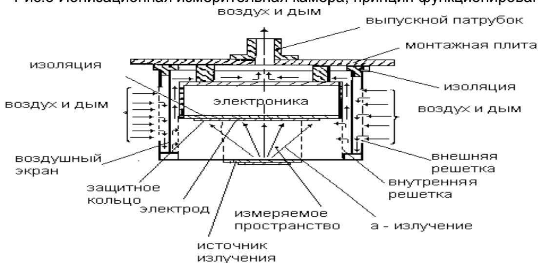
Рис.3 Ионизационная измерительная камера, принцип функционирования.
