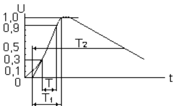
Кривая напряжения холостого хода (1,2/50 мкс)
